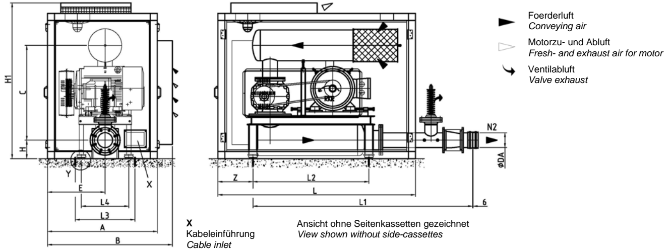
Detail Y Maschinenfuß Flexible socket
