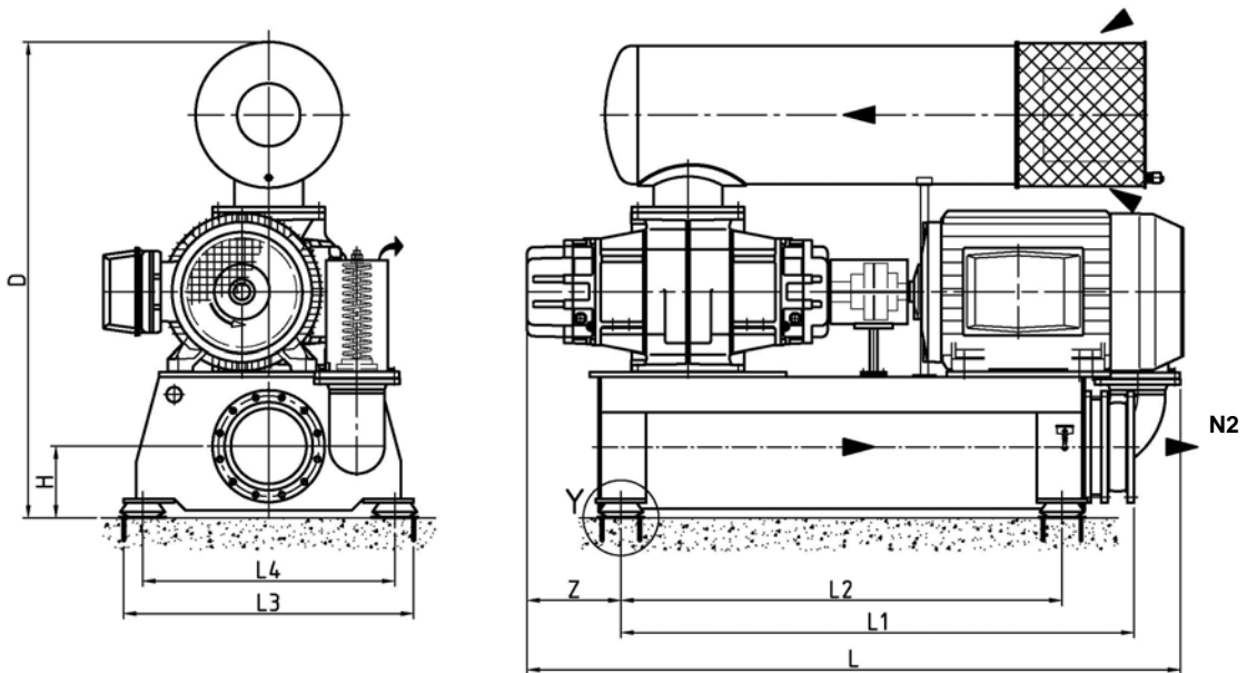
Detail Y Maschinenfuß Flexible socket
